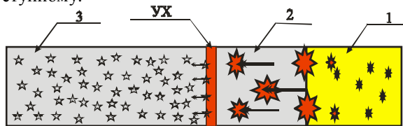
Рисунок 1 - Схема процесу детонації ЕВР україніт-ПП-1: 1-зона хімічної реакції; 2-стислий шар ЕВР; УХ-ударна хвиля; 3-заряд ЕВР до початку реакції.
