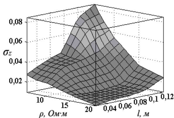
Рисунок 4 – Залежність \sigma_z = F(l[n], \rho[n])
