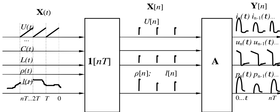
Рисунок 1 – Структурна схема електровибухового перетворення енергії
