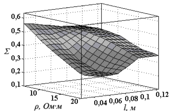
Рисунок 3 – Залежність M\Sigma[n]=F(I[n], \rho[n])
